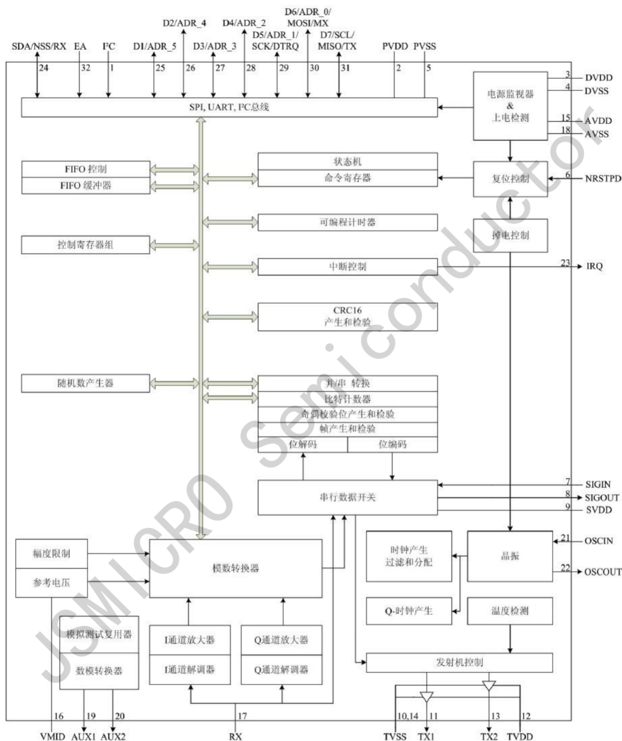
图 2 功能框图
