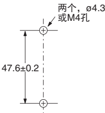
安装孔
