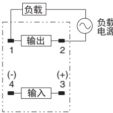
端子排布/内部连接 (顶视图)
