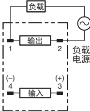
端子排布/内部连接 (顶视图)
