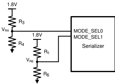
图 8-12. MODE_SEL[1:0] 连接图
