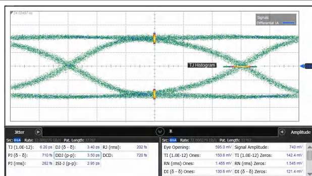
图 6-4. 32 Gbps 800 mV PRBS15 Source (1 dB Loss)
