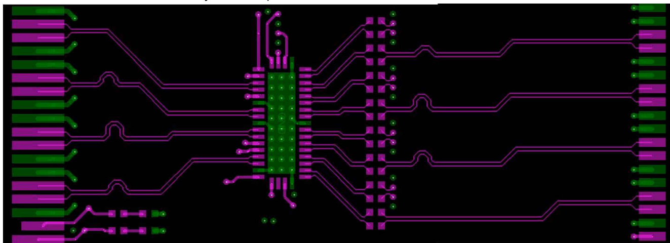
图 10-1. SN75LVPE5421 Layout Example
